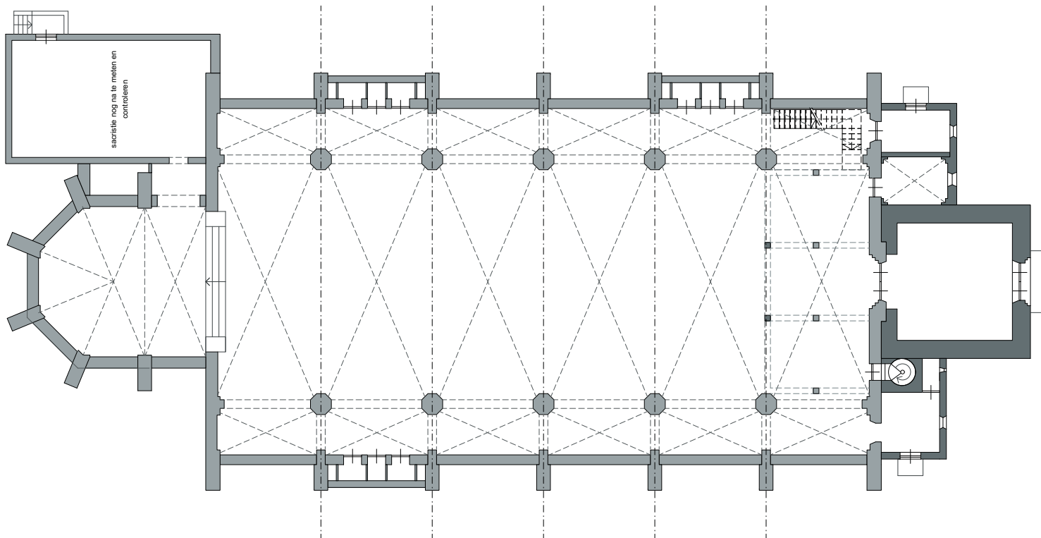
Plattgrond huidige kerk
